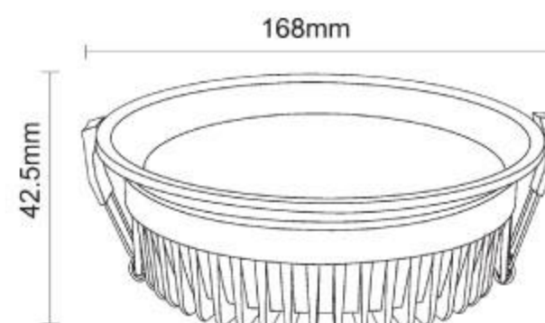
Cut-Out D158mm
