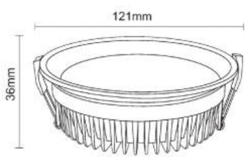
Cut-Out D112mm
