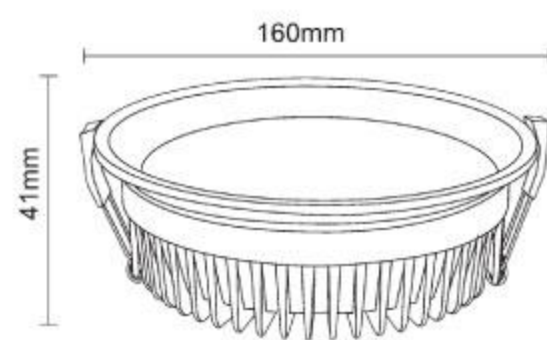
Cut-Out D150mm
